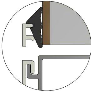
Detalj dräneringshål
