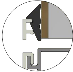
Detalj dräneringshål
