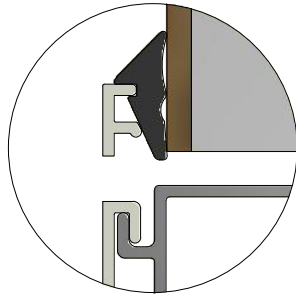
Detalj dräneringshål
