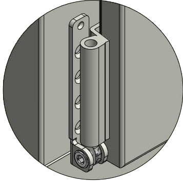
Detalj gångjärn
