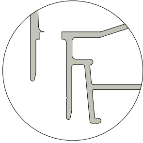
Dräneringshål
