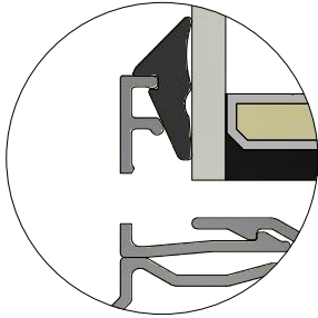
Dräneringshål
