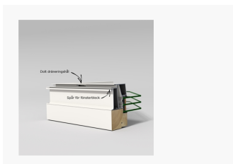
Montering av fönsterbleck LF11283 Royal. Dräneringshålen sitter undertill. Fönsterblecket monteras i det inre spåret, innanför dräneringshålet.
